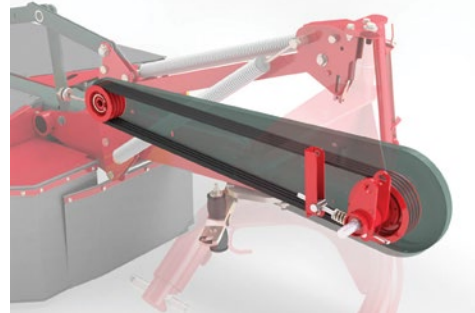
Amortiguador de golpes.
